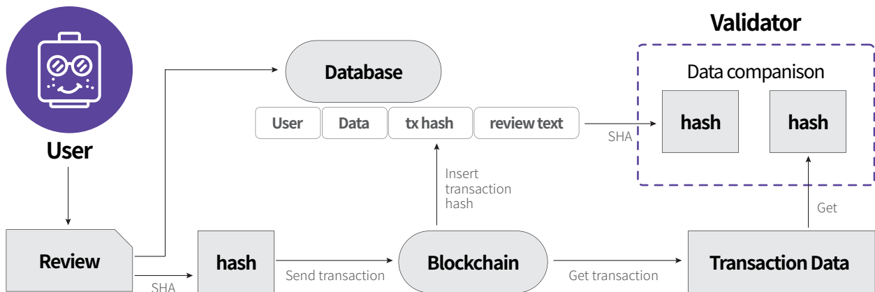
Fig. 13. Data Validation
