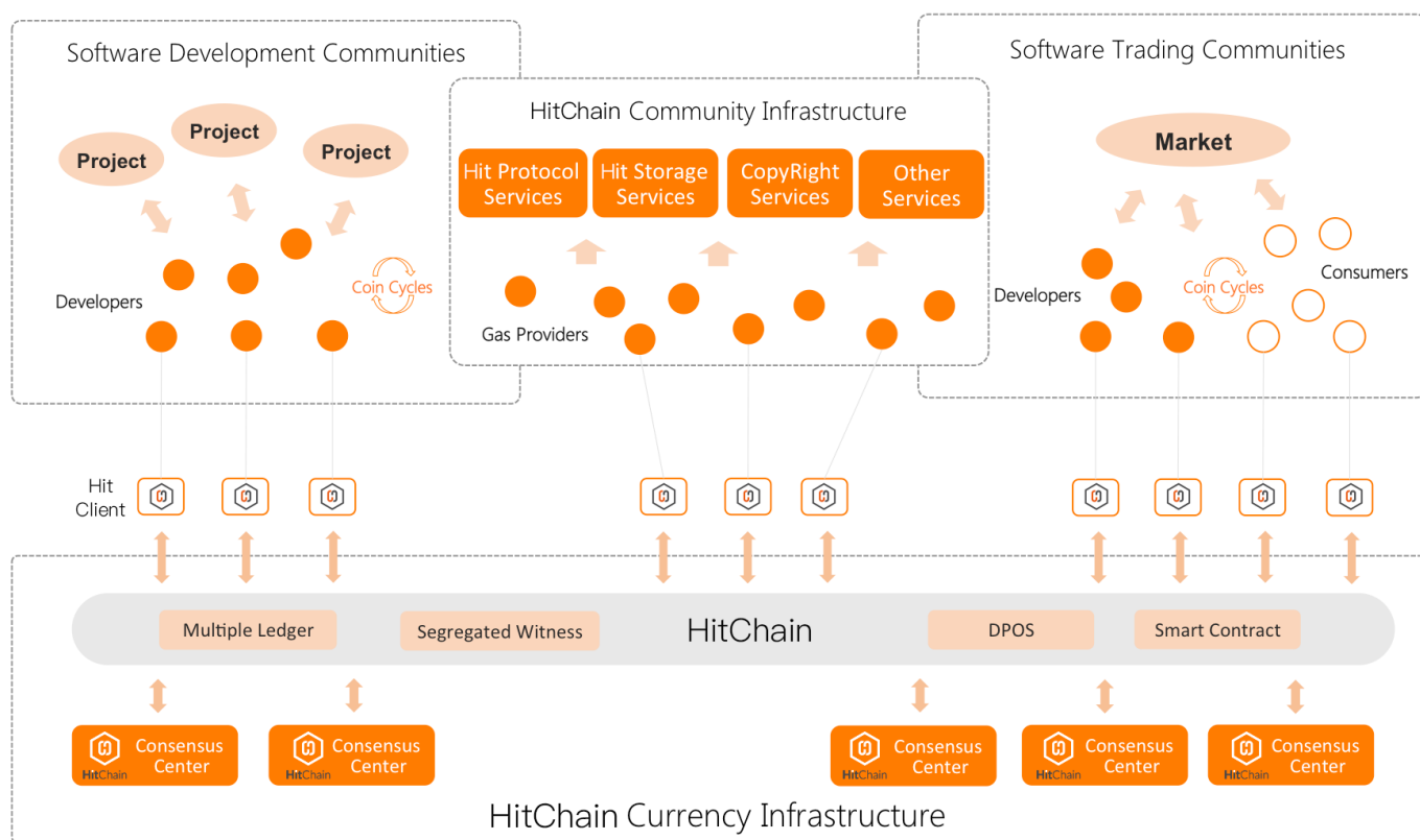
HitChain生态系统结构图
