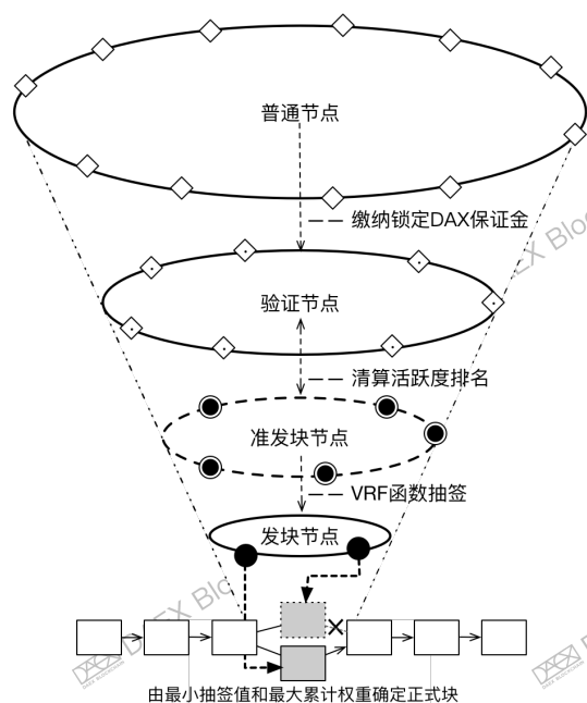
图 15: ASPOS 的区块创建过程
