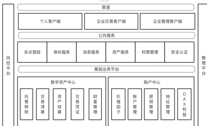
图 11：多资产钱包产品结构
